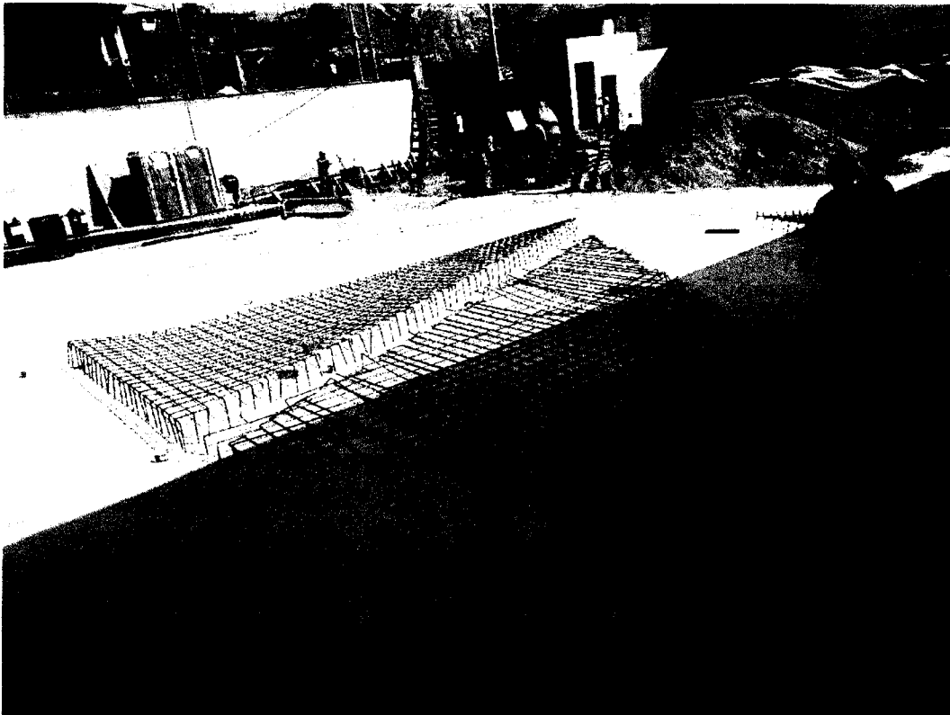
FOTO N° 02: Habilitación de acero para malla de rampa de ingreso.
